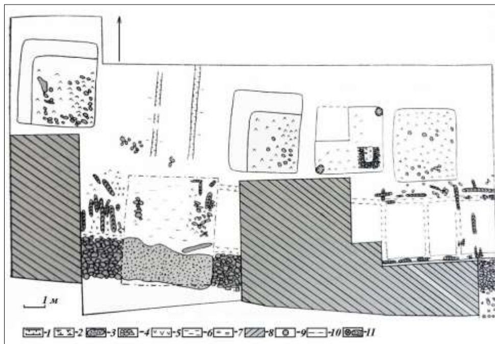
Рис. 3. План розкопу в'їзної вежі на дитинці в Ревно
