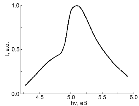
Рис. 4. Спектр збудження люмінесценції тонких плівок ZnGa_2O_4 , відпалених у вакуумі.
