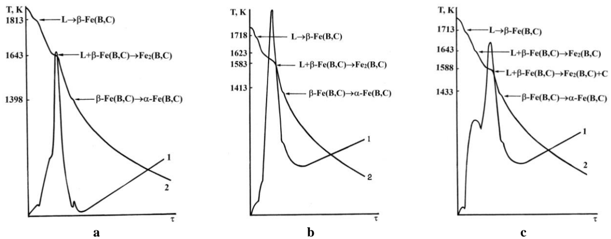
Fig. 2. Thermograms of Fe – 12.1 % B – 0.1 % C (a), Fe – 10.8 % B – 0.3 % C (b), Fe – 11.0 % B – 1.24 % C (c) alloys: 1 – \Delta T(\tau) ; 2 – T(\tau) .
