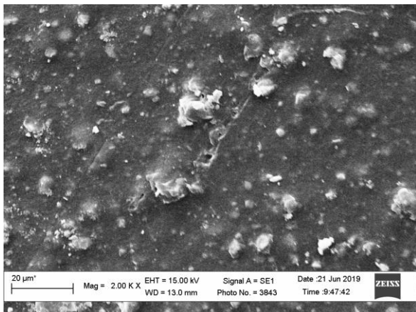
Рис. 12. Зростання дефектності поверхні поліетиленової плівки із наповнювачем Sredolen (23,2 ваг. %) на 7 рік складування. X 2000
