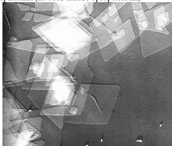
Рис. 16. Мікрофотографія лінійного поліетилену, вирощеного із розчину тетраліну за температури 89 °С. Зображення надане Dr. R. V. Rice [6].
