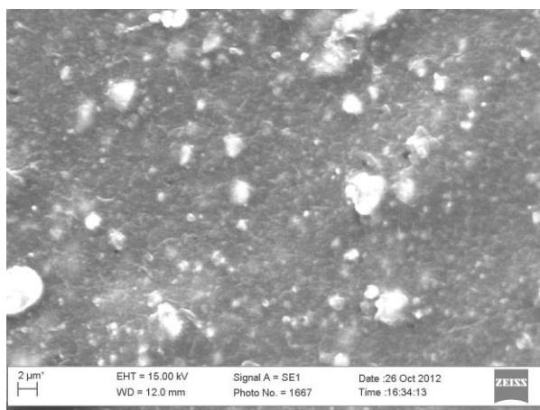
Рис. 5. Структура поверхні поліетиленової плівки змішаним наповнювачем Vatpol (22,6 ваг. %): X 2000.
